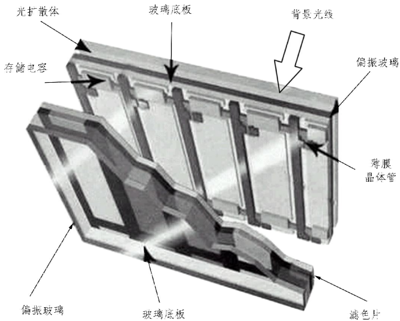
图 4-1 LCD 屏的结构
